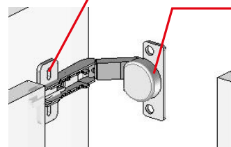
Folding door hinge
